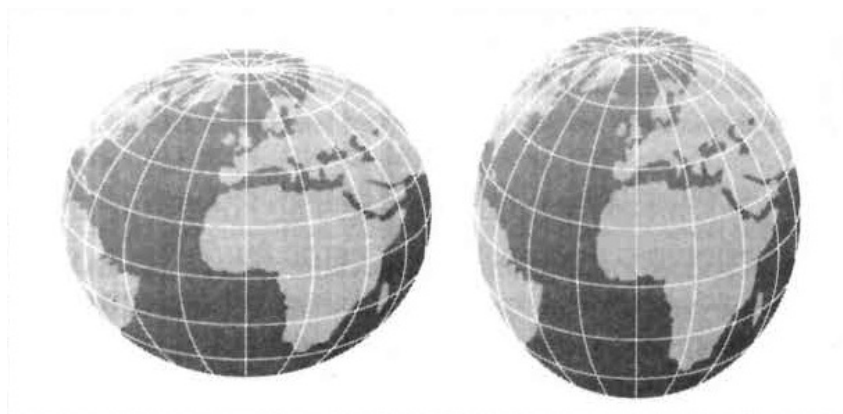
A la izquierda, la Tierra newtoniana, con forma de sandía, y a la derecha, la Tierra cartesiana, con forma de melón.
