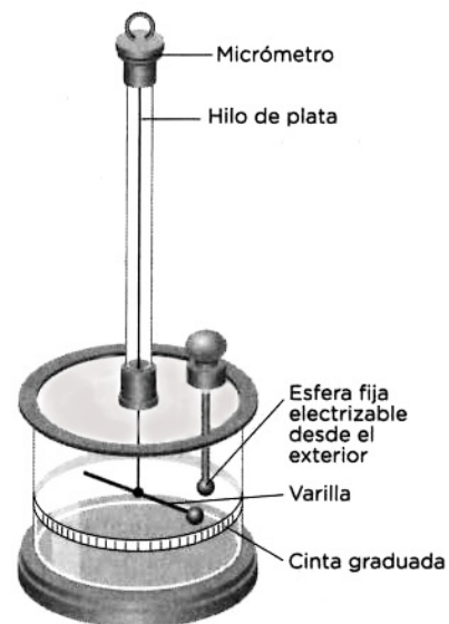
La balanza de torsión de Coulomb.
