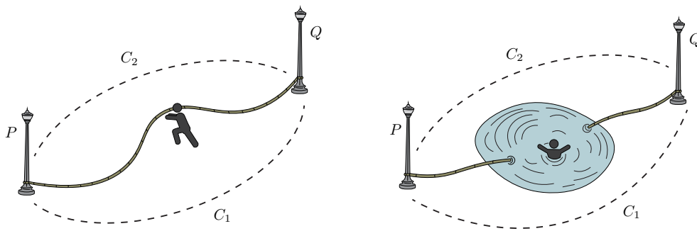
Figura 2: En (a) los caminos C_1 y C_2 son homotópicos. En (b), el camino C_1 no se puede deformar continuamente en el camino C_2 . Fuente: Imagen elaborada por Raymundo Iván González Ballesteros (basada en [Ku93, p.39]).
