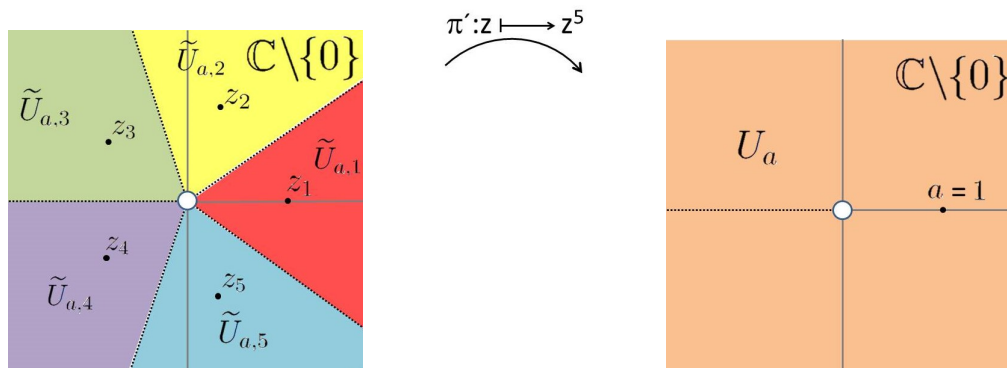
Figura 1: El espacio cubriente asociada a la raíz quinta. La fibra sobre a = 1 es el conjunto \pi^{-1}(a) = \{z_1, z_2, z_3, z_4, z_5\} de raíces quintas de la unidad. La imagen inversa bajo \pi del abierto U_a = \mathbb{C} \setminus \{z \in \mathbb{C} : \operatorname{Re}(z) \leq 0, \operatorname{Im}(z) = 0\} es la unión disjunta de las “rebanadas” \tilde{U}_{a,1}, \tilde{U}_{a,2}, \tilde{U}_{a,3}, \tilde{U}_{a,4} y \tilde{U}_{a,5} .
