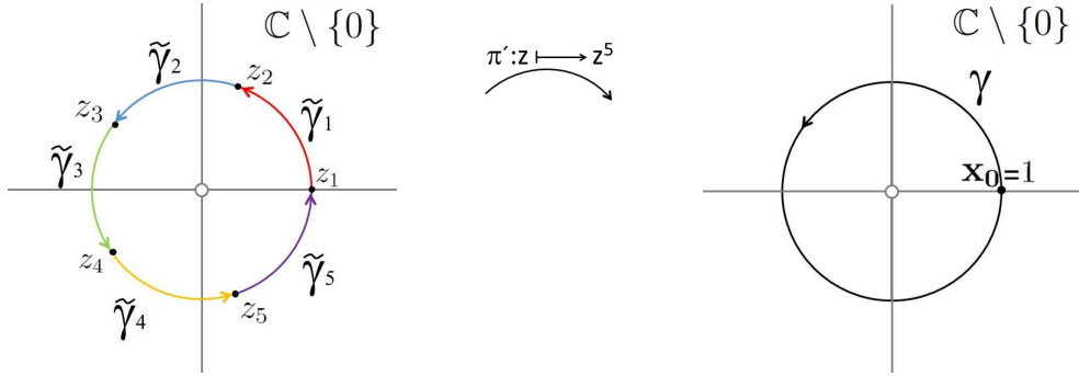
Figura 3: Levantamientos \tilde{\gamma}_1, \tilde{\gamma}_2, \tilde{\gamma}_3, \tilde{\gamma}_4 y \tilde{\gamma}_5 del lazo \gamma basado en \mathbf{x}_0 = 1 en el espacio cubriente \pi' : \tilde{X} \rightarrow X asociado a la raíz quinta.
