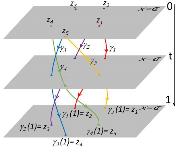
Figura 4: Un lazo de polinomios \gamma basado en \mathbf{x}_0 = (z_1, z_2, z_3, z_4, z_5) corresponde a una trenza.
