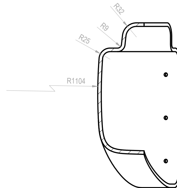
A-A (1:5)
