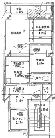
1 层平面图
