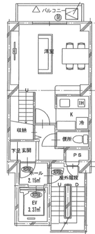
6 层平面图
