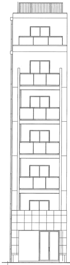
北側立面图
