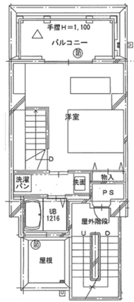
7 层平面图
