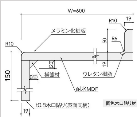
■カウンター断面図
